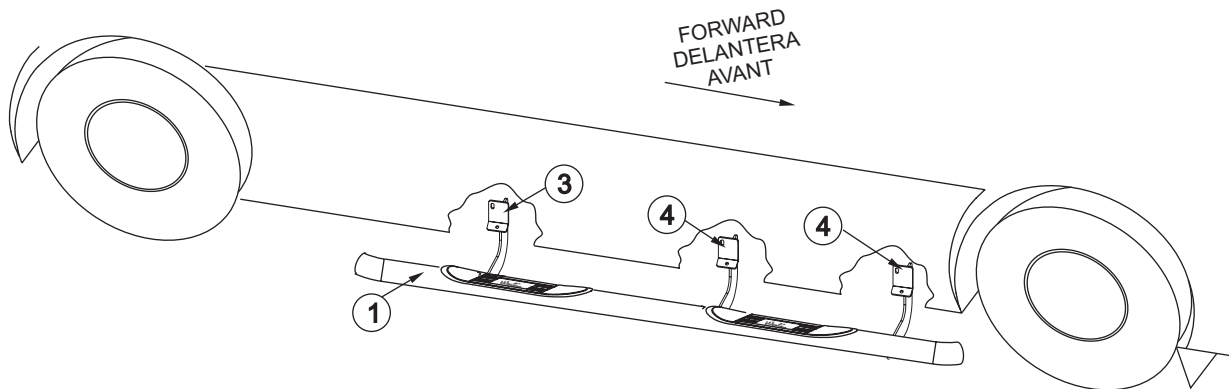
FIGURE 1 INSTALLATION VIEW OF PASSENGER SIDE SHOWN, DRIVERS SIDE OPPOSITE FIGURA 1 VISTA DE LA INSTALACIÓN DEL LADO DEL CONDUCTOR OPUESTO AL LADO DEL ACOMPAÑANTE FIGURE 1 ILLUSTRE: COTE CONDUCTEUR, EN FACE: COTE PASSAGER
