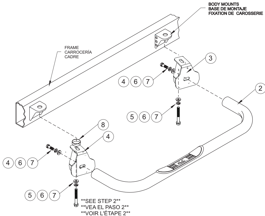
FIGURE 1 INSTALLATION VIEW OF DRIVER SIDE SHOWN, PASSENGER SIDE OPPOSITE FIGURA 1 VISTA DE LA INSTALACIÓN DEL LADO DEL CONDUCTOR OPUESTO AL LADO DEL ACOMPAÑANTE FIGURE 1 ILLUSTRÉ: CÔTÉ CONDUCTEUR, EN FACE: CÔTÉ PASSAGER
