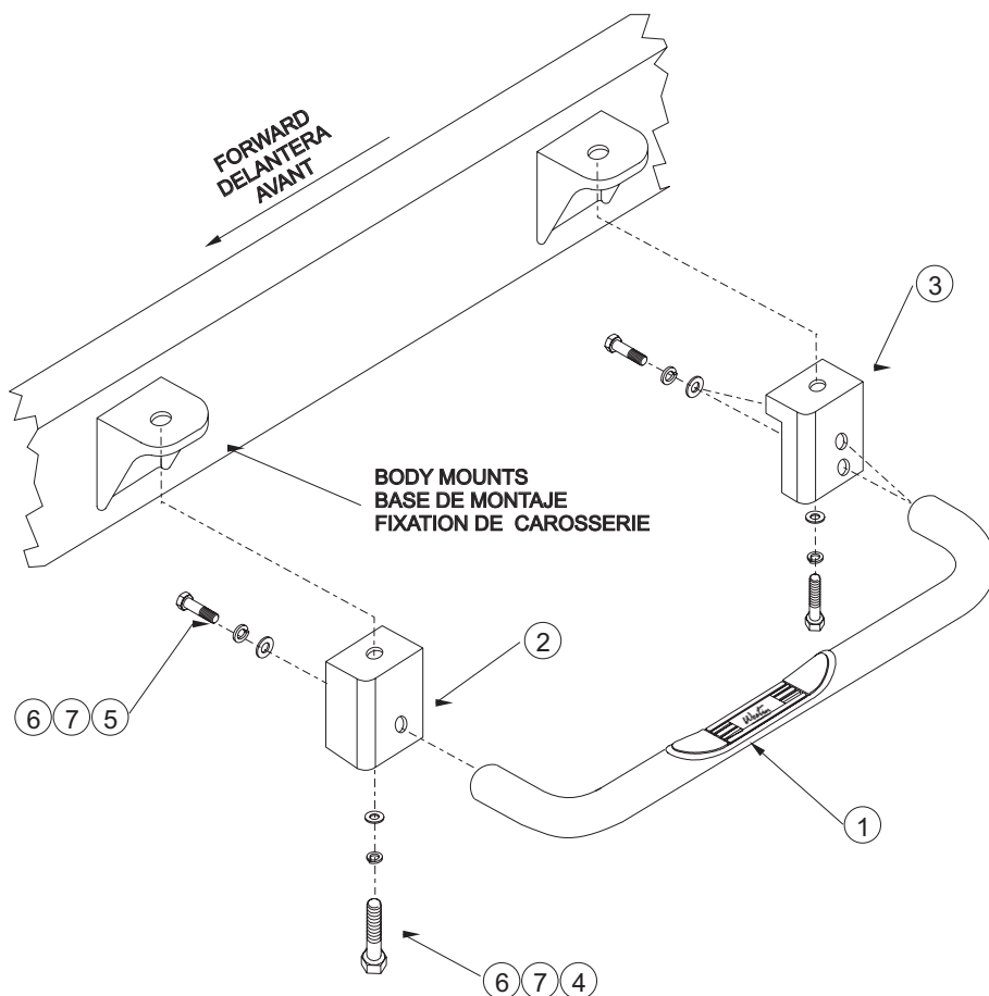
INSTALLATION VIEW OF DRIVER SIDE SHOWN, PASSENGER SIDE OPPOSITE VISTA DE LA INSTALACIÓN DEL LADO DEL CONDUCTOR OPUESTO AL LADO DEL ACOMPAÑANTE ILLUSTRE: COTE CONDUCTEUR, EN FACE: COTE PASSAGER
