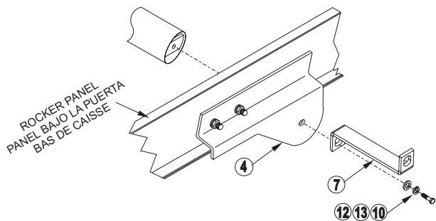
FIGURE 1 COTE CONDUCTEUR CABINE REGULIERE
