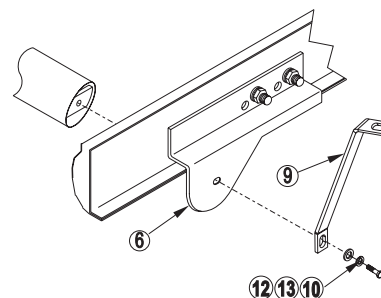
FIGURE 2 COTE CONDUCTEUR CABINE RALLONGÉE ARRIERE
